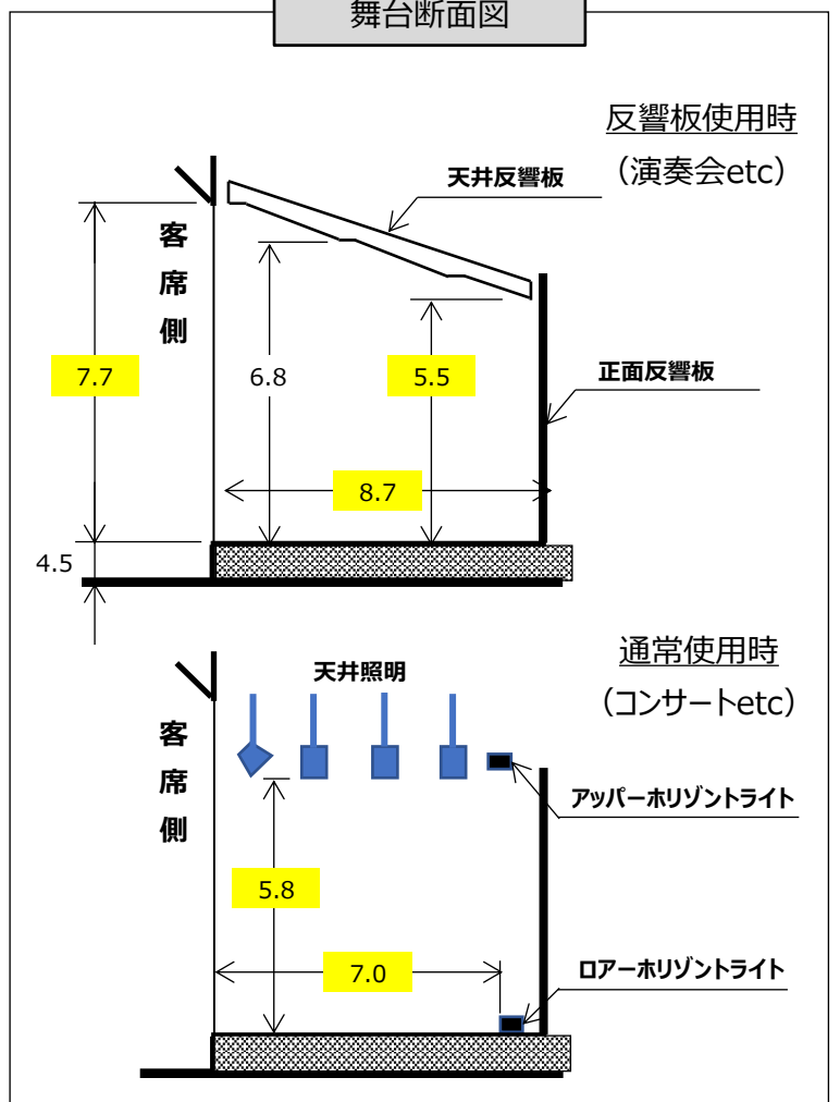
舞台断面図
